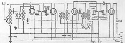
Diagrama del circuito "Contrafase", en el que se puede ver cómo están dispuestos los condensadores tandem y las bobinas toroidales.
